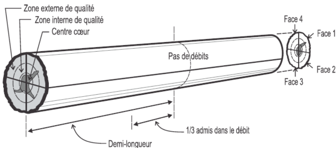
Figure 57 Délimitation des débits : défauts à la découpe
