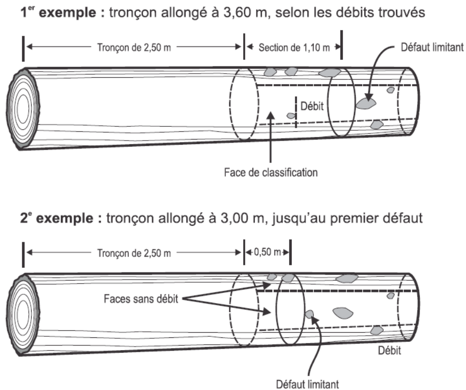
Figure 66 Procédure pour allonger un tronçon selon les débits
