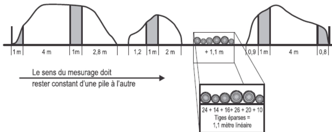
Figure 78 Délimitation des segments de piles à mesurer et à dénombrer
