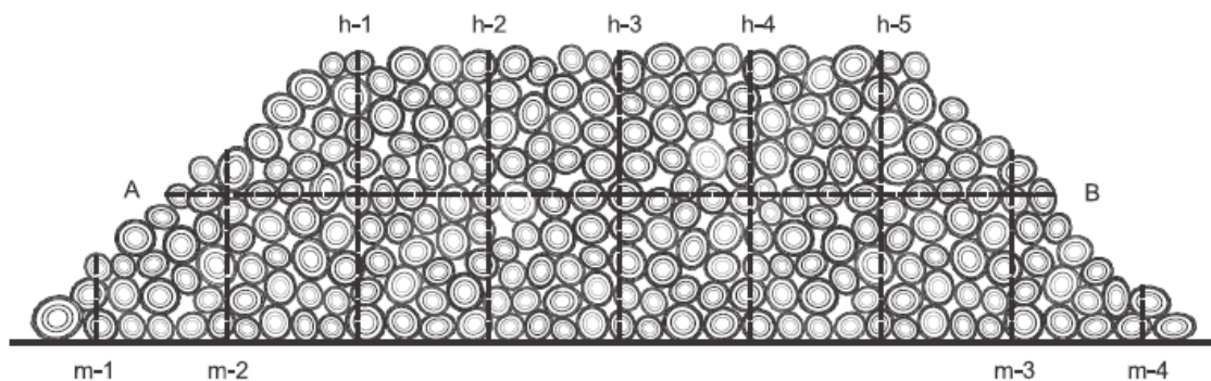
Figure 41 Longue pile régulière, sans supports latéraux
