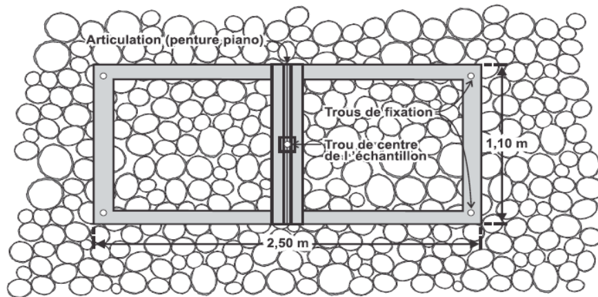
Figure 71 Gabarit pour un échantillon rectangulaire
