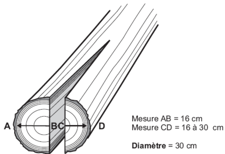
Figure 14 Mesurage d'une découpe avec fente ouverte
